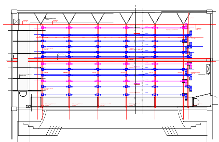
GRONDPLAN TROMMELTREKKEN
